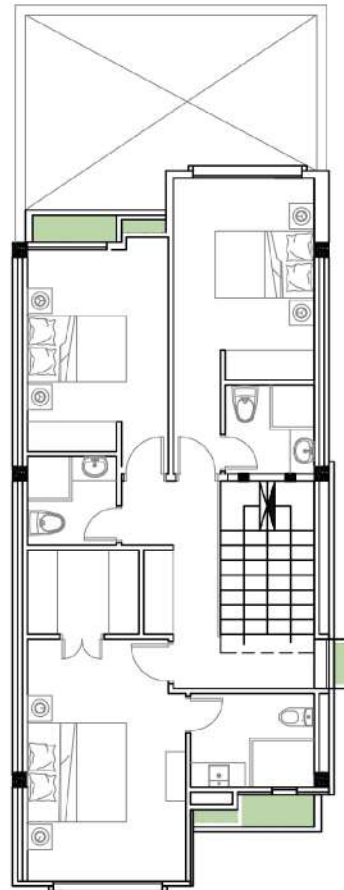
PLANTA ALTA
